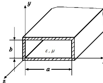
图 1 矩形波导
